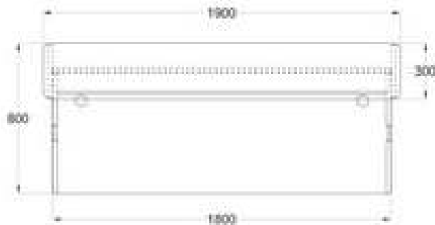
PIS 16 - 1600 (W) X 800 (D) X 1200 (H) PIS 19 - 1900 (W) X 800 (D) X 1200 (H)
